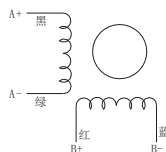
接线图
