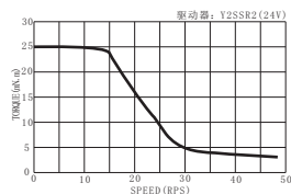
力矩曲线图
